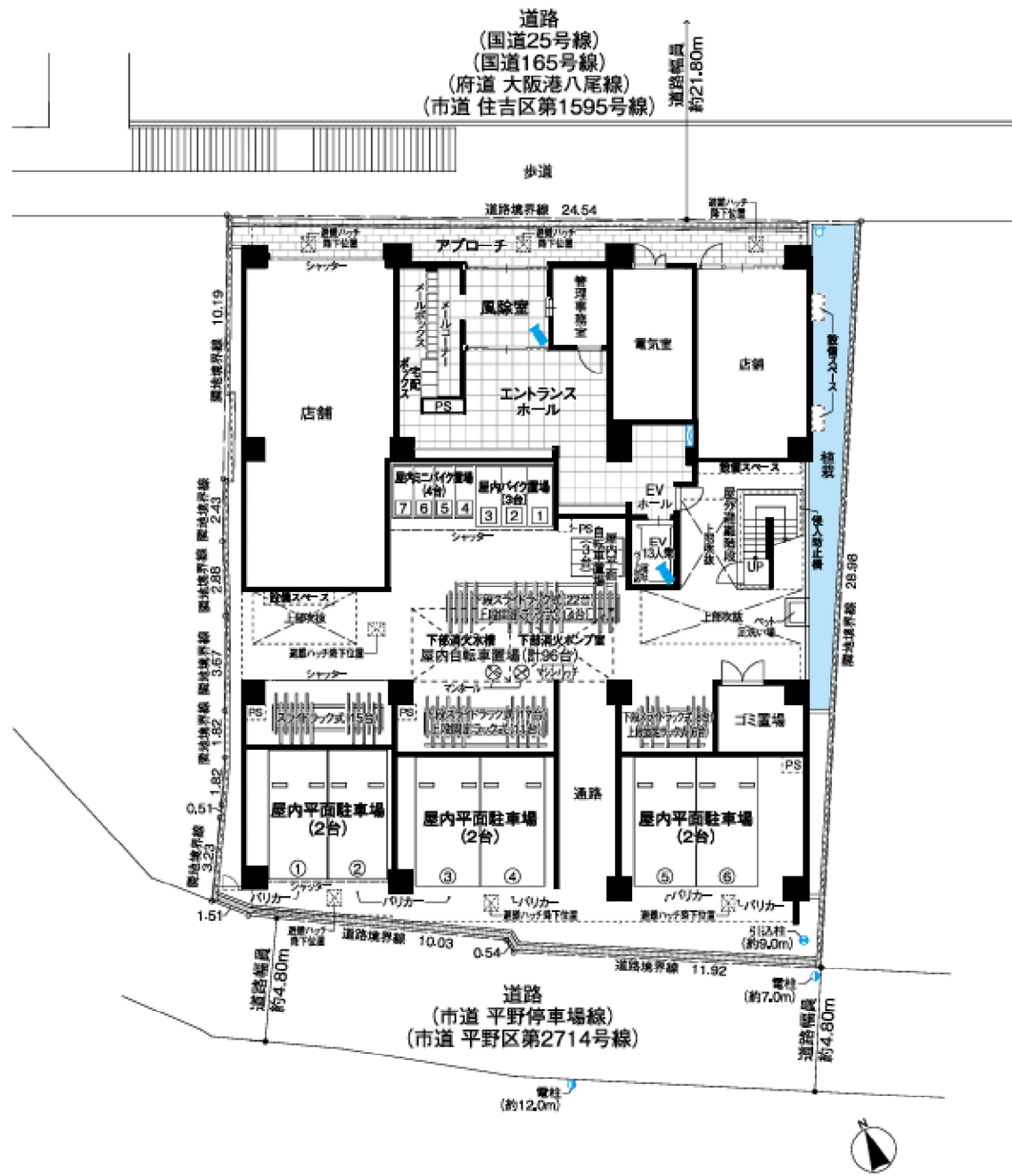
◇敷地配置図・1階平面図 scale 約1/300
