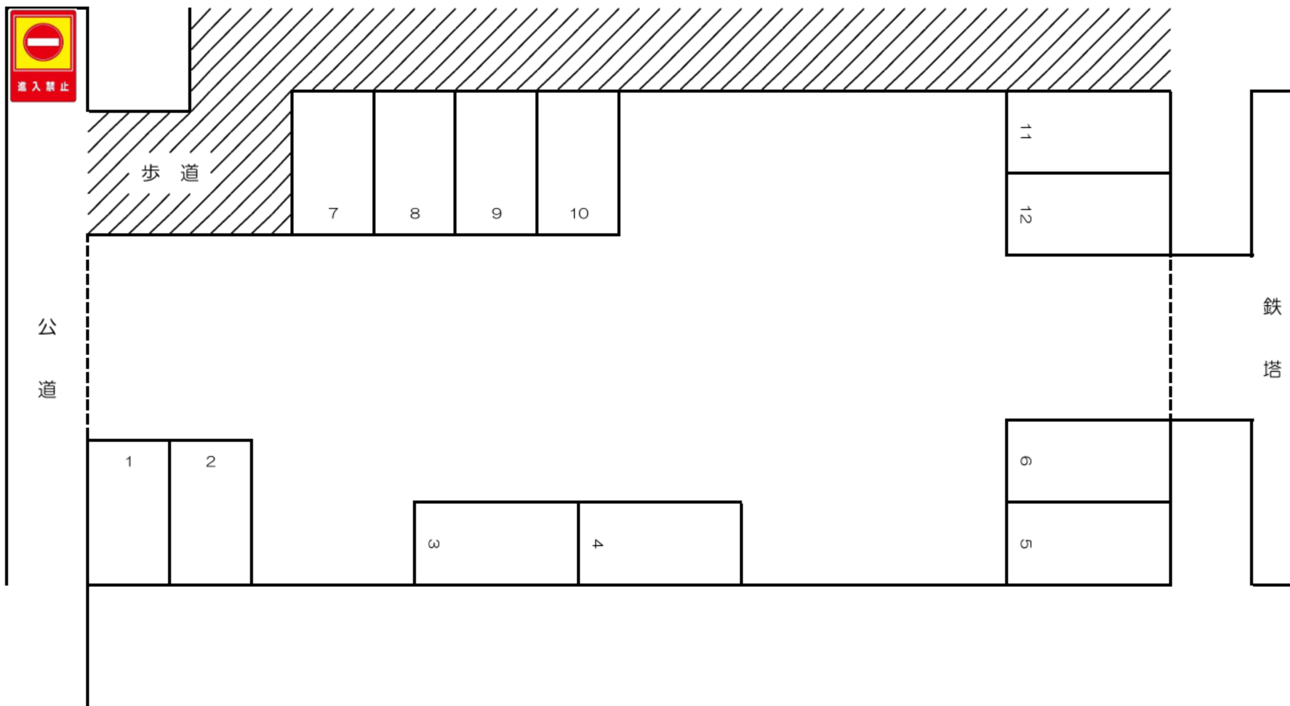
木場第4駐車場配置図
