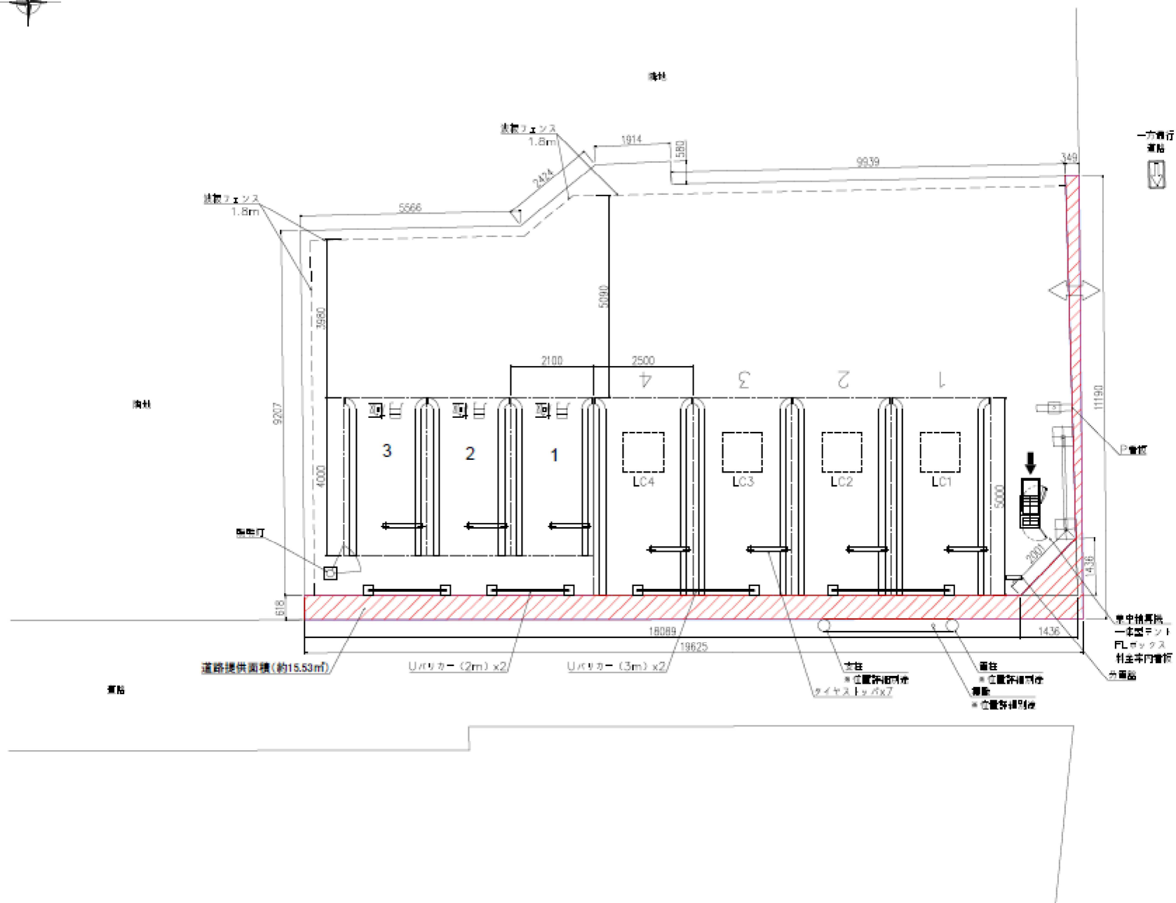
平面図 (S=1:50)
