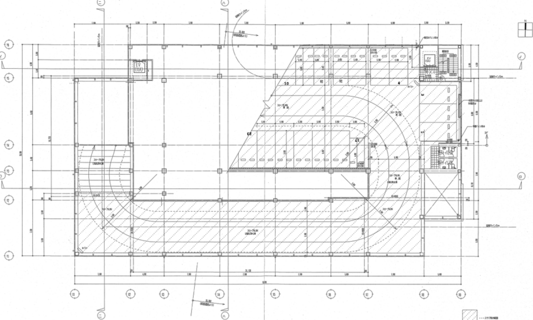
30層平面図
