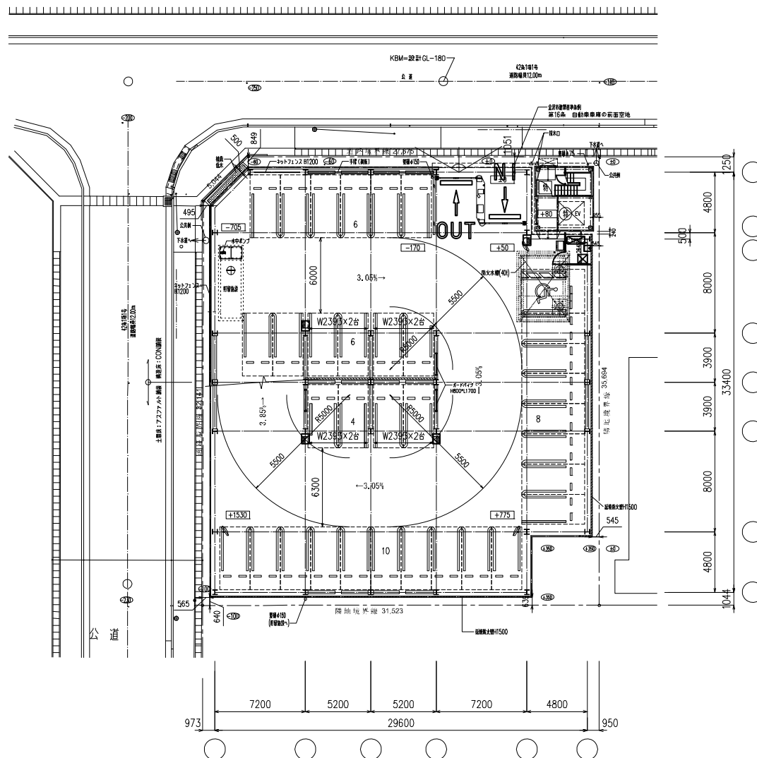
配置図・1階平面図
