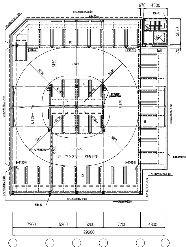
4階平面図
