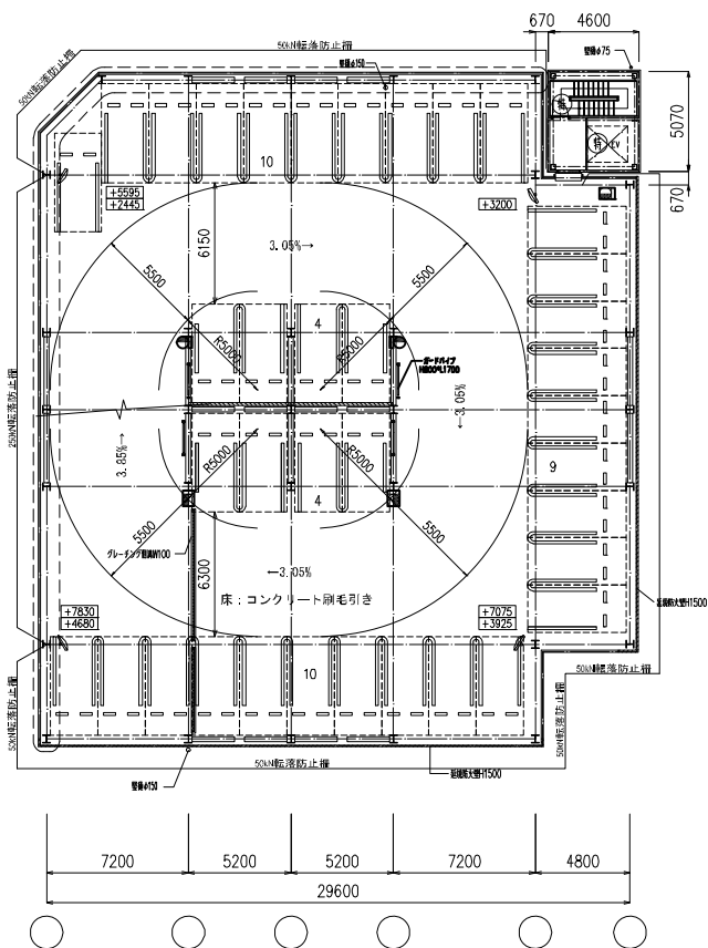
2階-3階平面図
