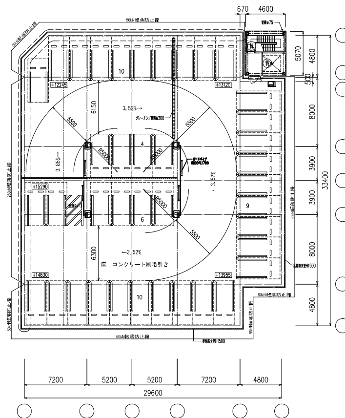
R階平面図
