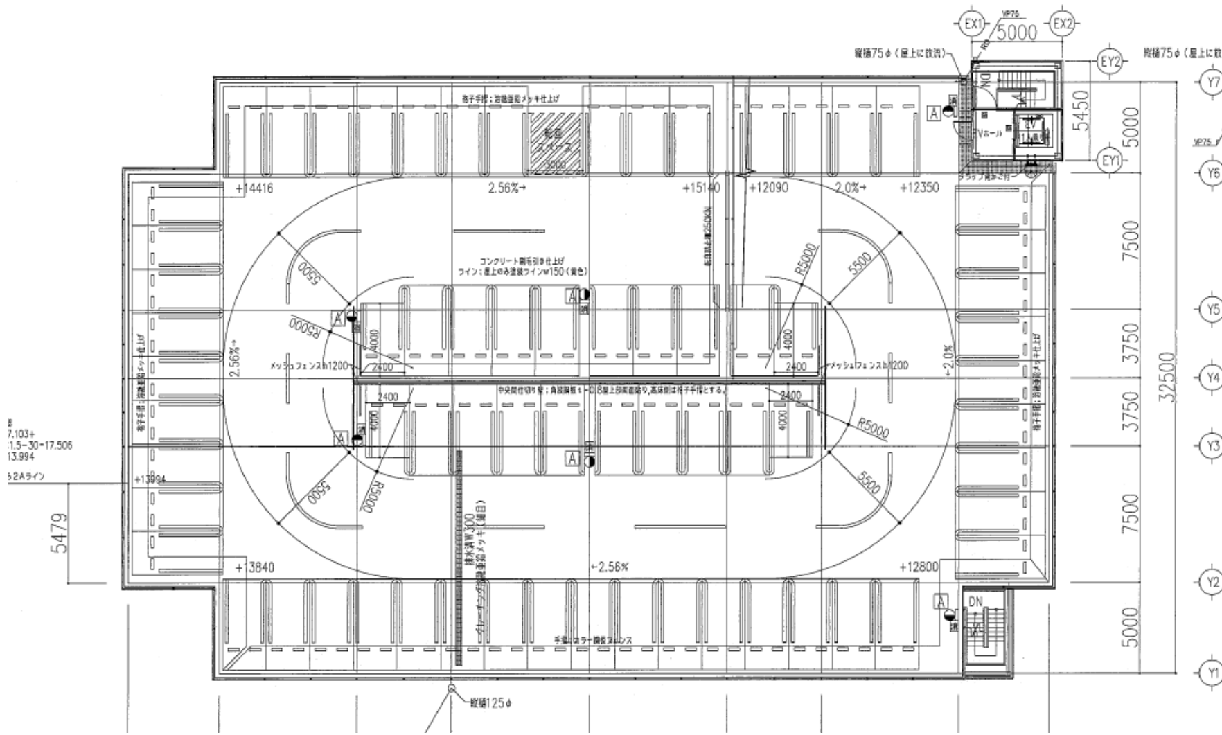
屋上階平面図
