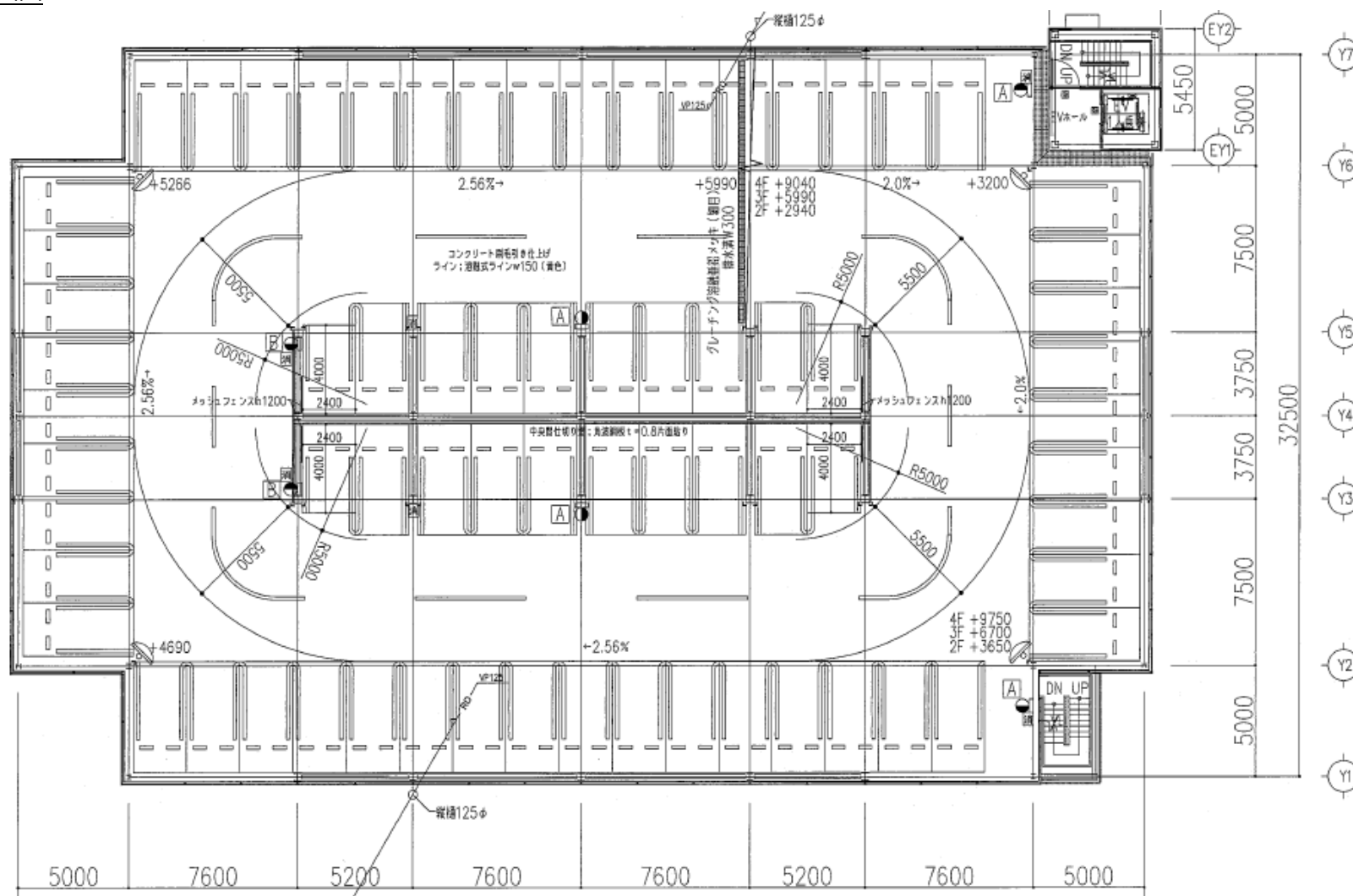
4 階平面図
