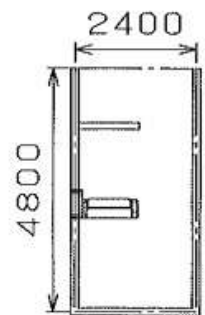
車室寸法
