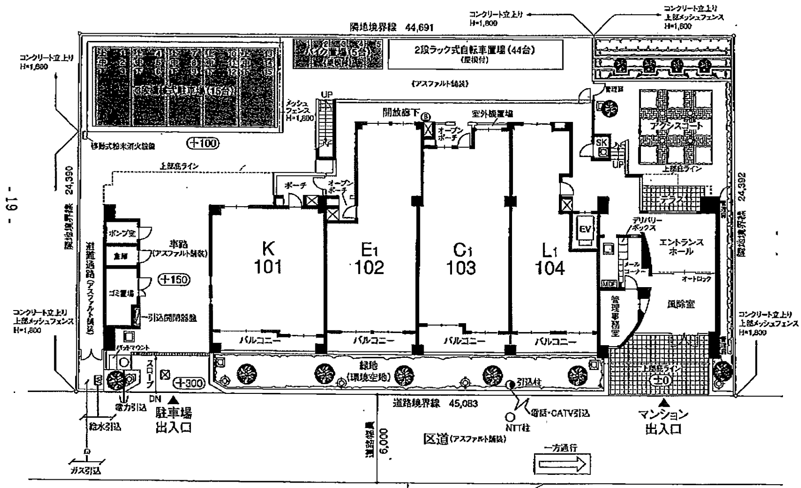
敷地配置図・1階平面図
