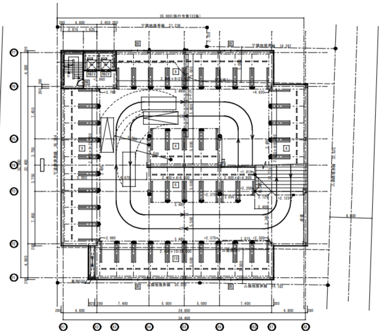
2階平面図 1/200
