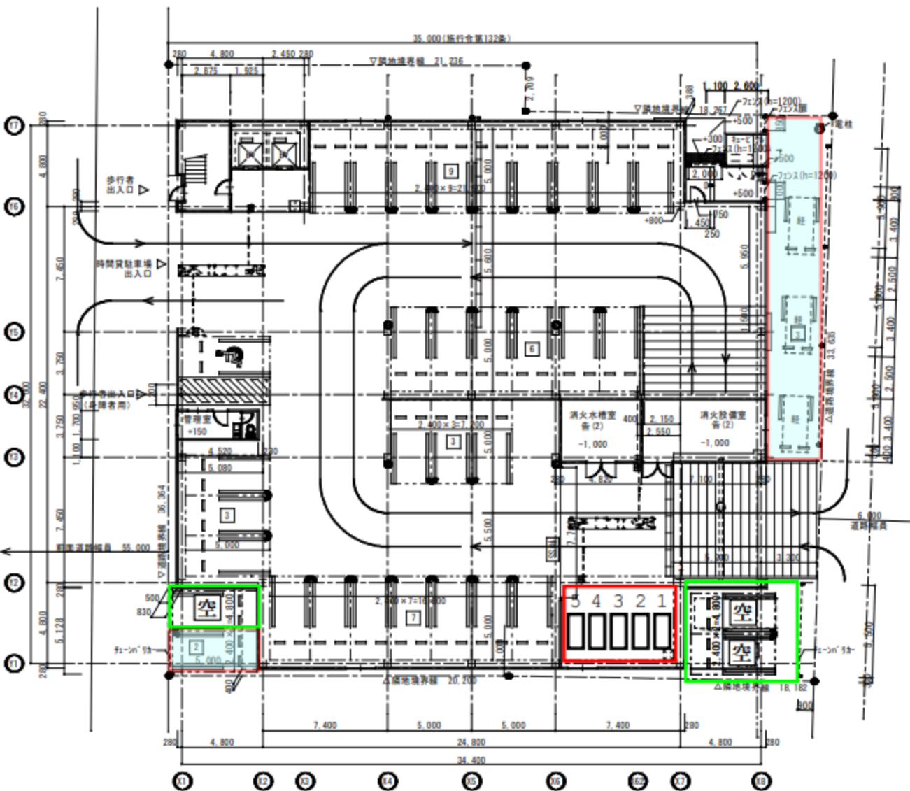
1階平面図 1/200
