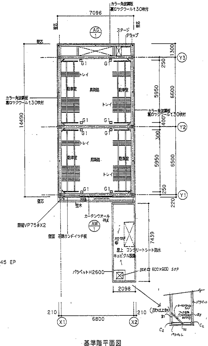
基準階平面図
