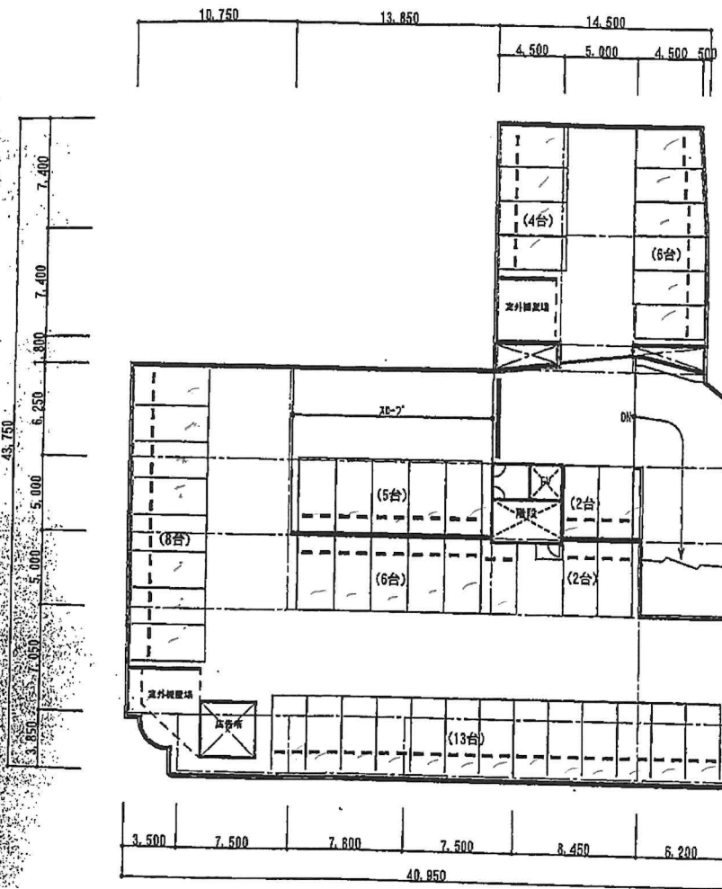
R階平面図 S=1/300
