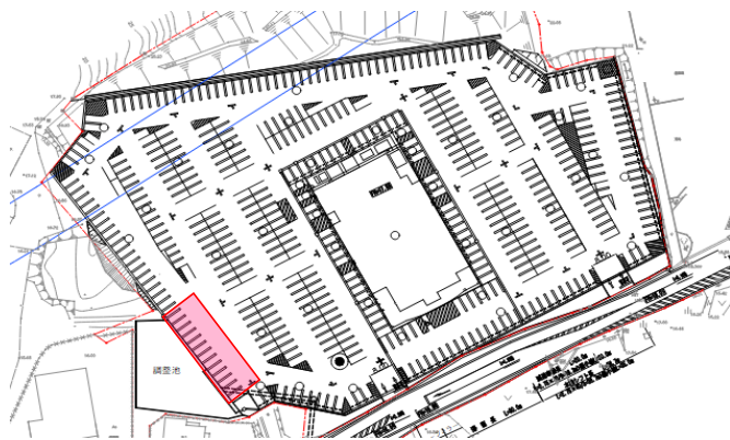
全体図
