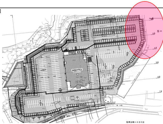
全体図
