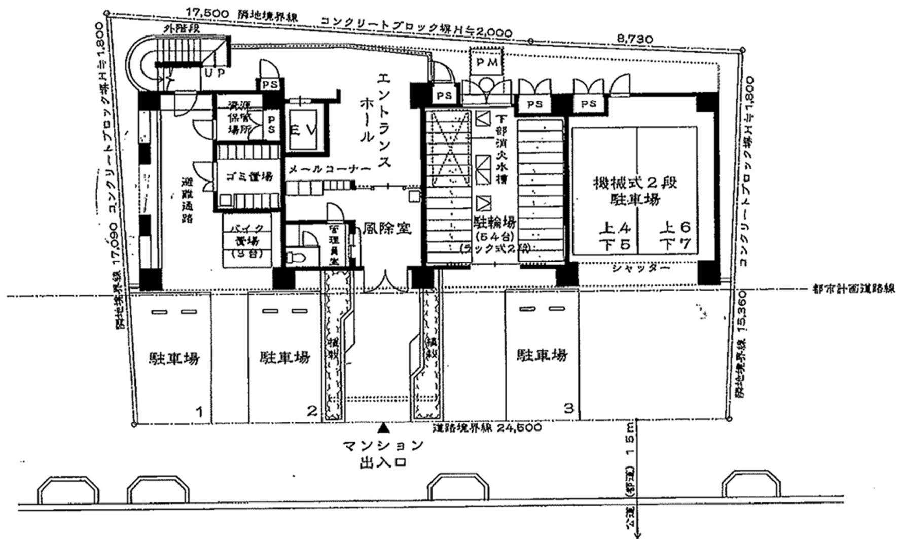
敷地配置図・1階平面図
