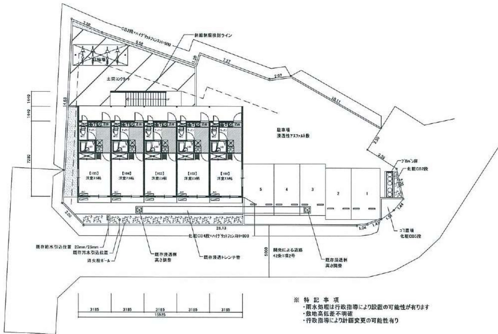
【 平面計画図 1/200 】
