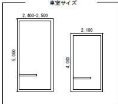
車室サイズ
