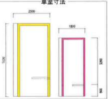
車室寸法
