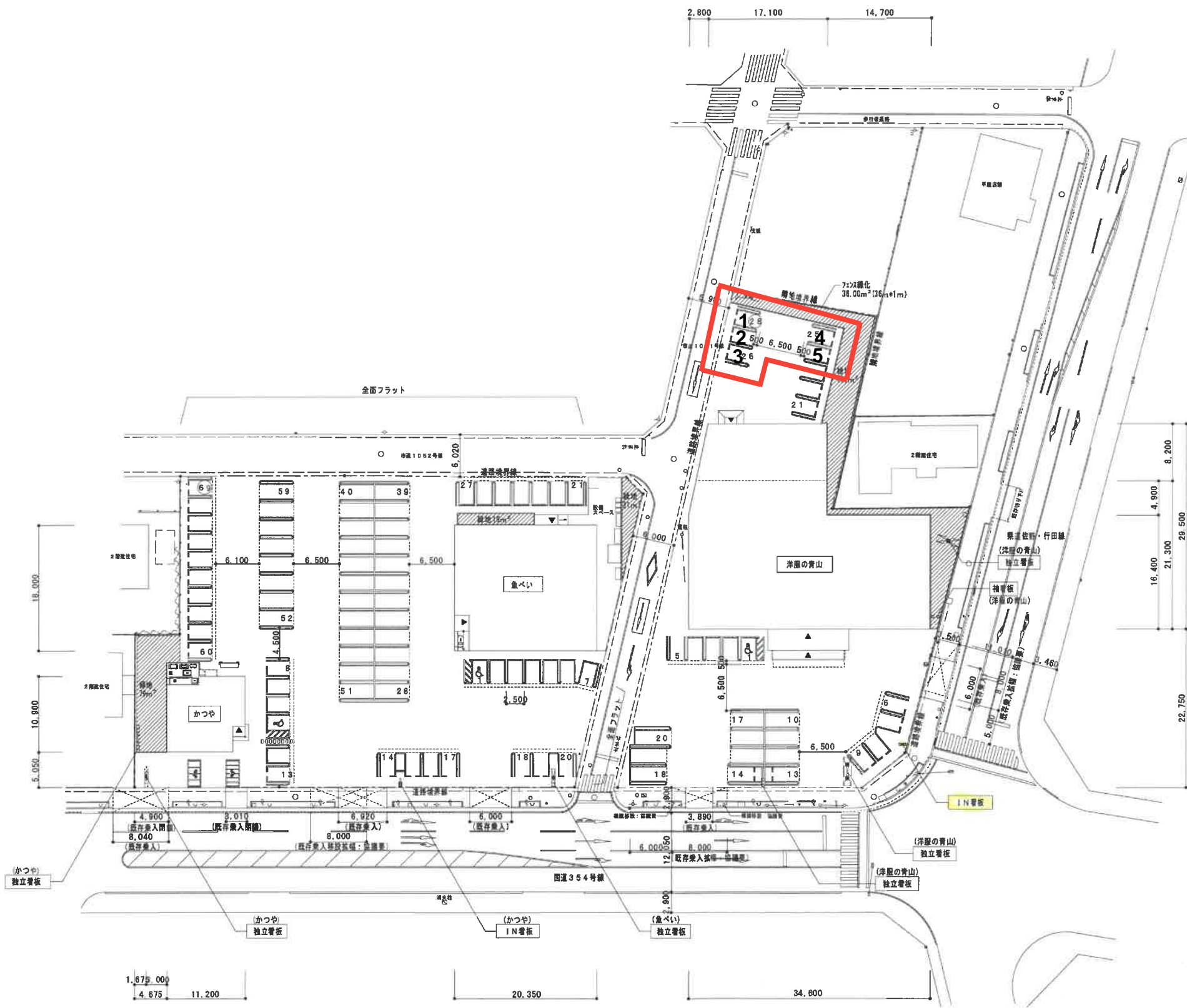
配置図 1:400
