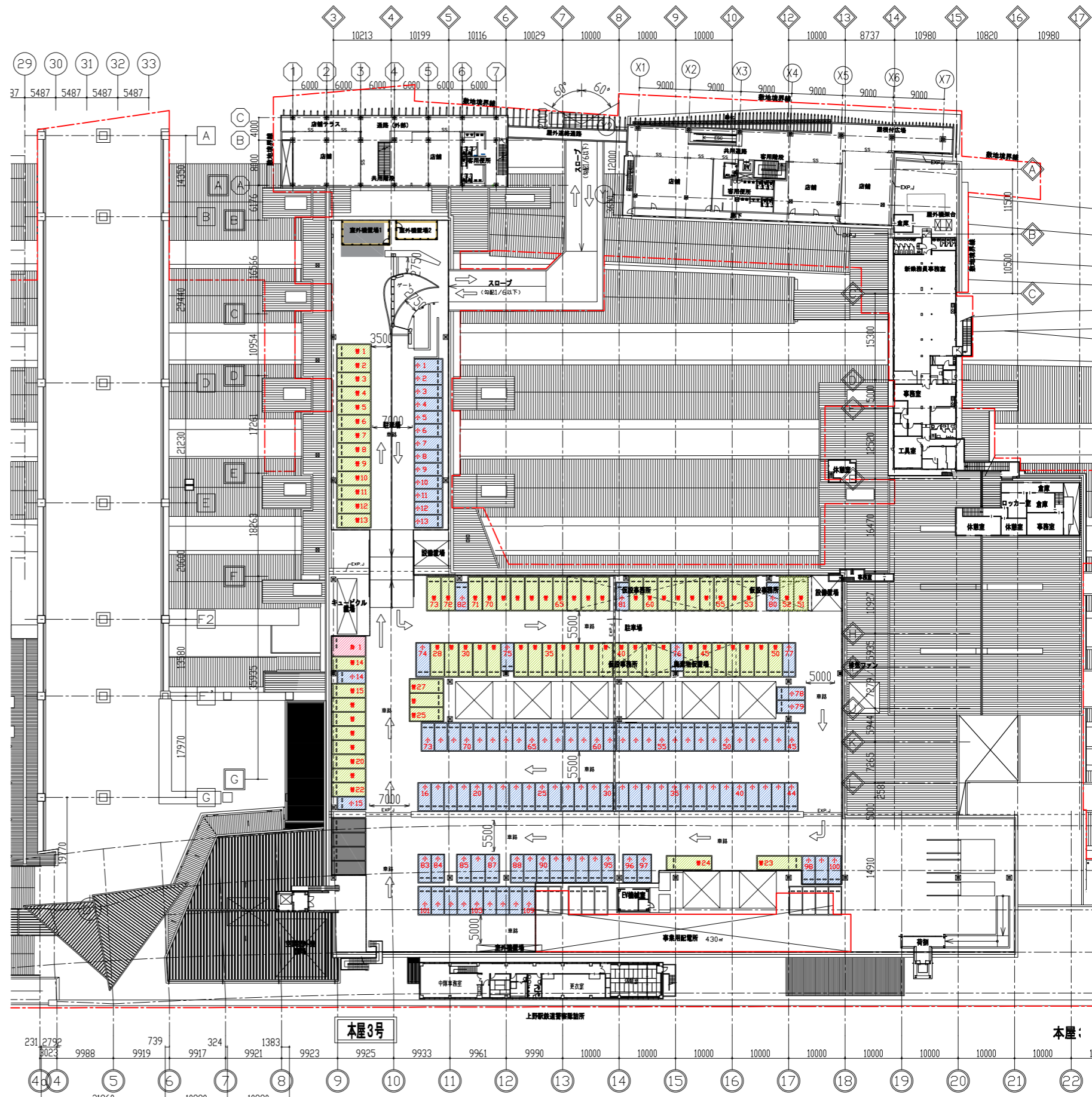
5階平面図
