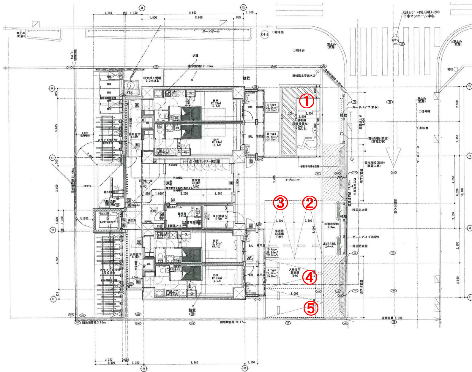
1階平面図
