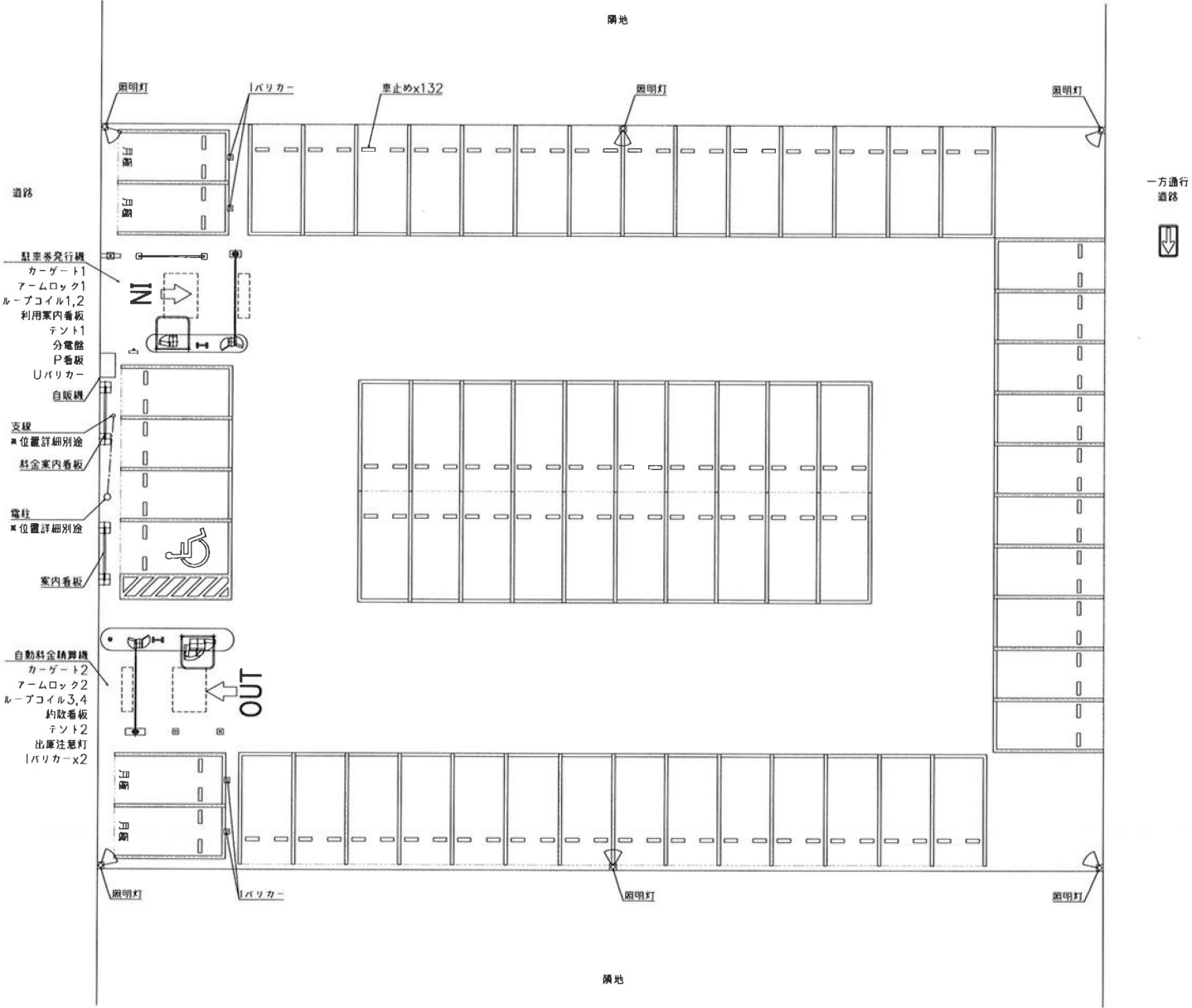
平面図 (S=1:100)
