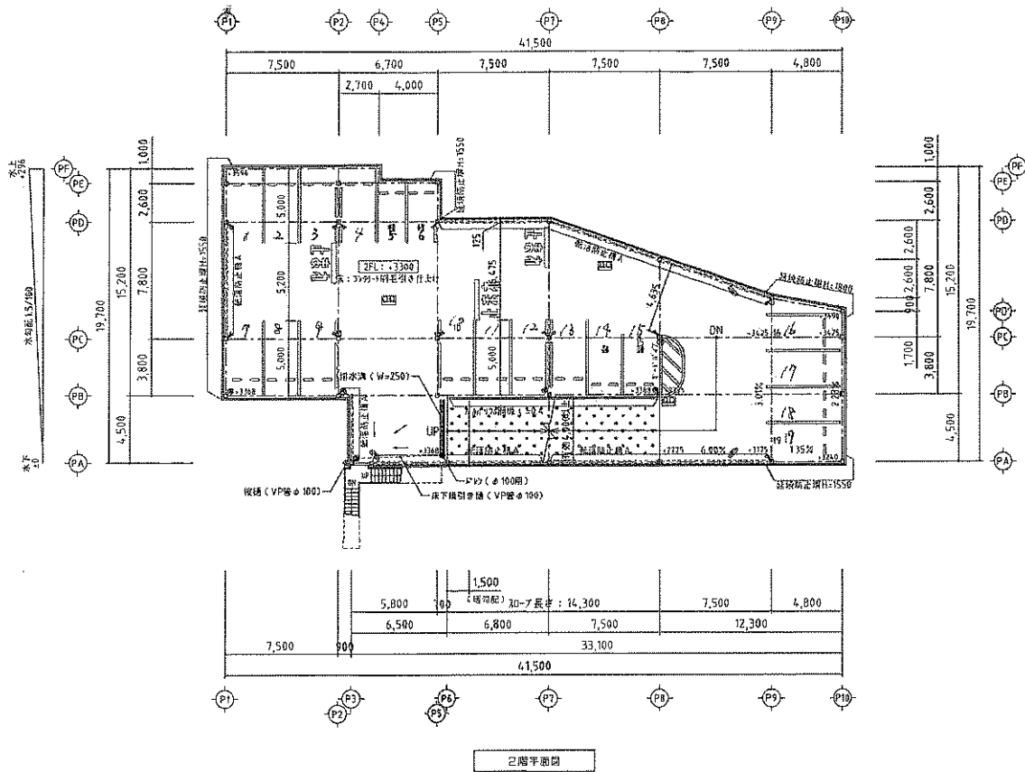
2階平面図
